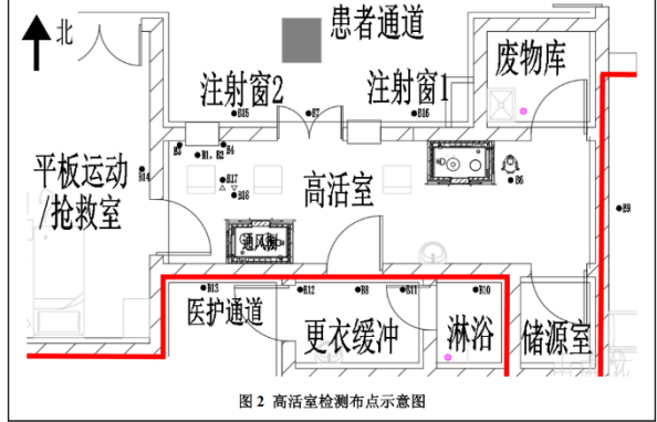
图 2 高活室检测布点示意图
