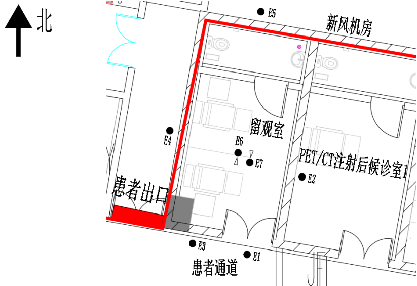
图 5 留观室检测布点示意图
