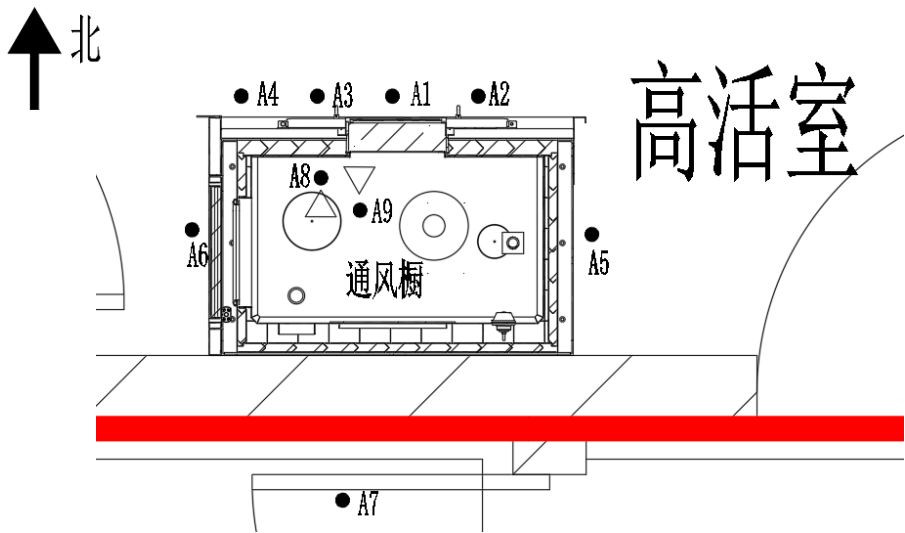
图 1 通风橱检测布点示意图
