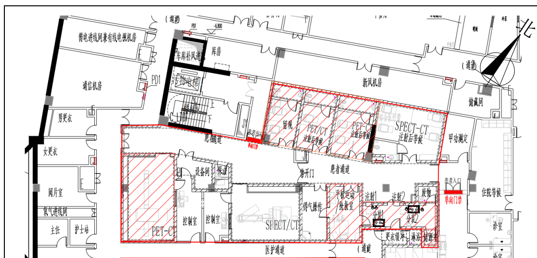
图 3-2 PET/CT 辐射工作场所平面布局示意图
