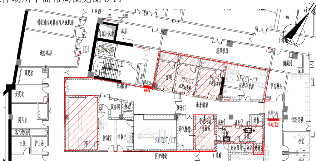
图 6-1 核医学科核素诊疗区 PET/CT 辐射工作场所平面布局图
